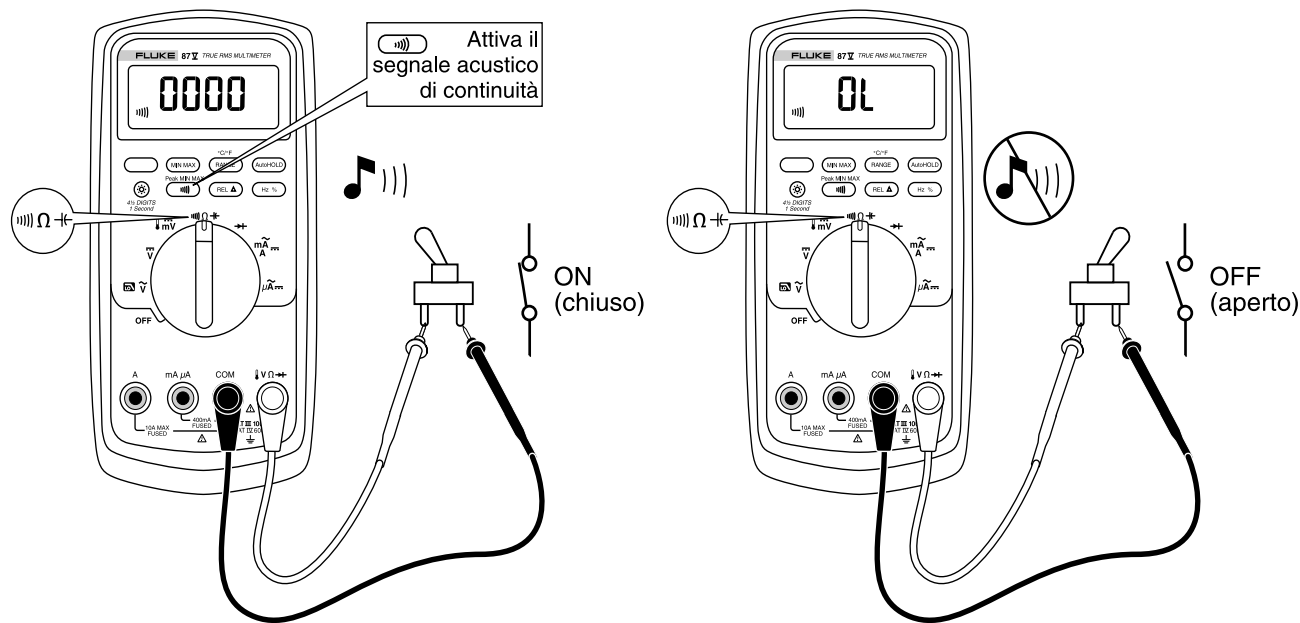
Figura 4. Prove di continuità
