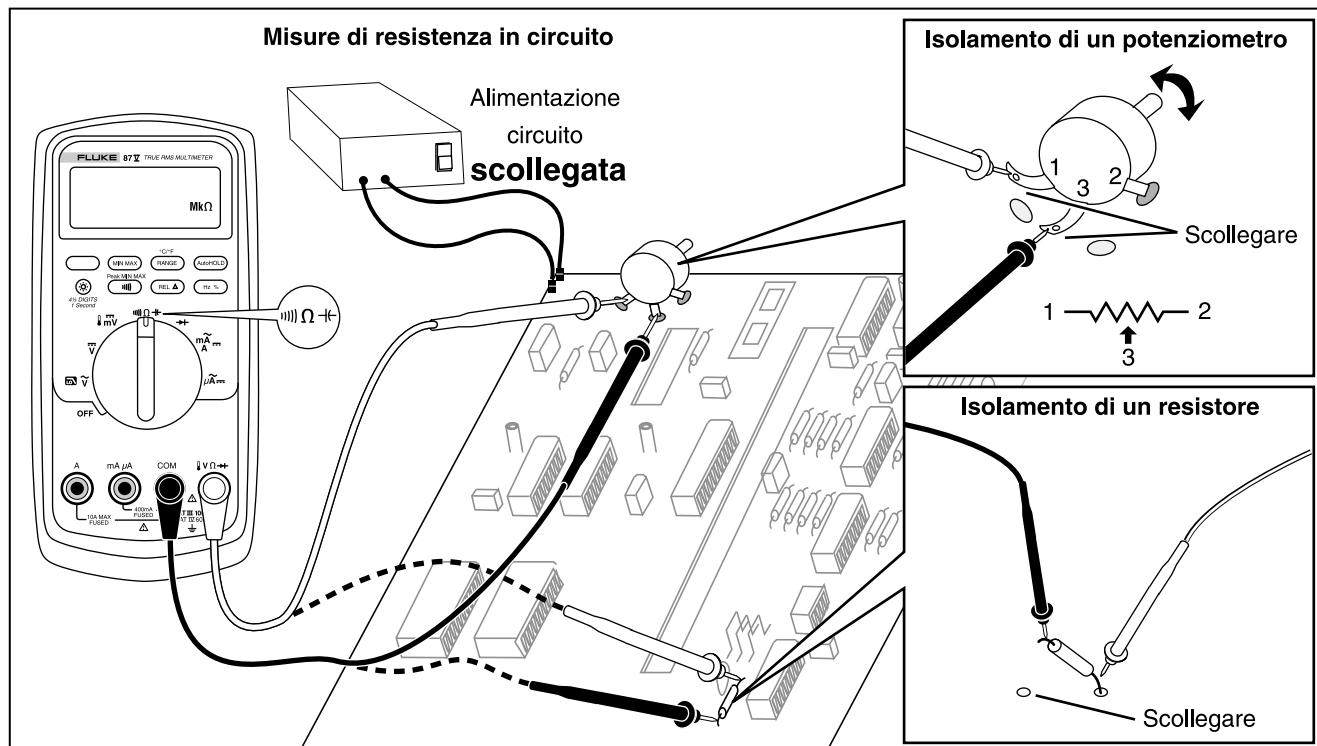
Figura 5. Misura di resistenza
