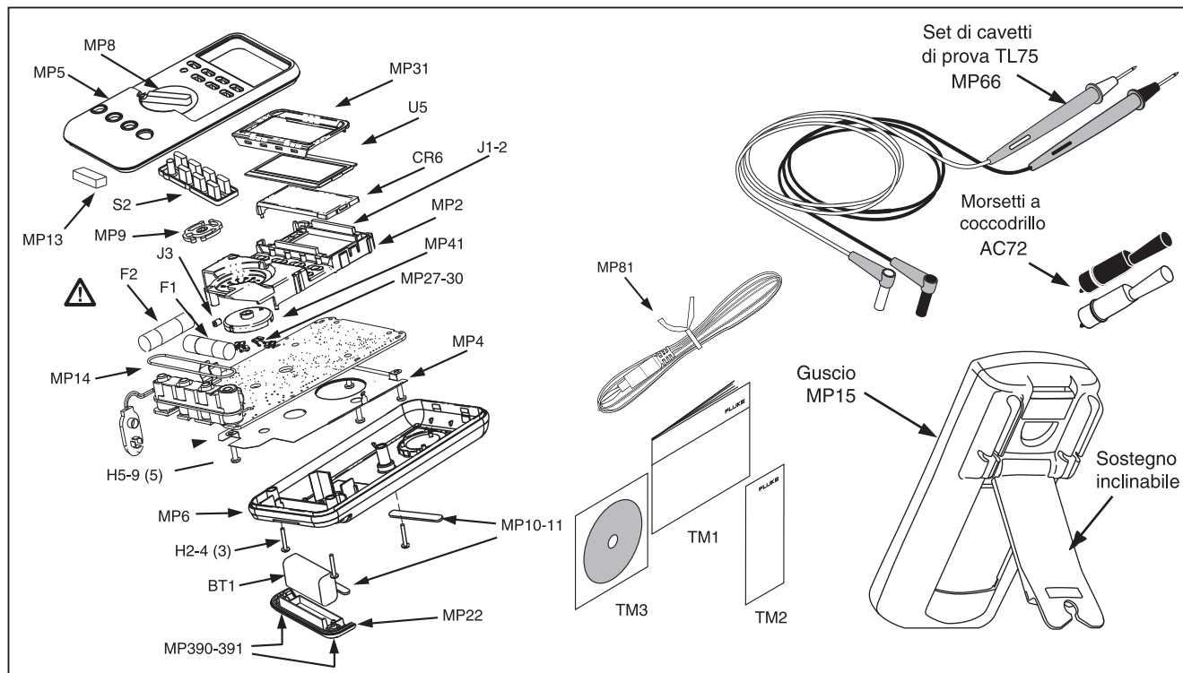
Figura 12. Parti sostituibili
