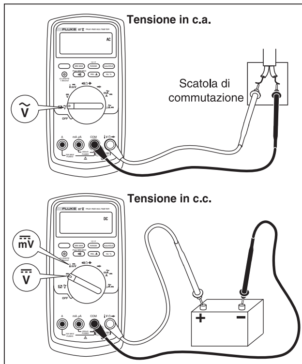
Figura 2. Misure di tensione in corrente alternata e continua
