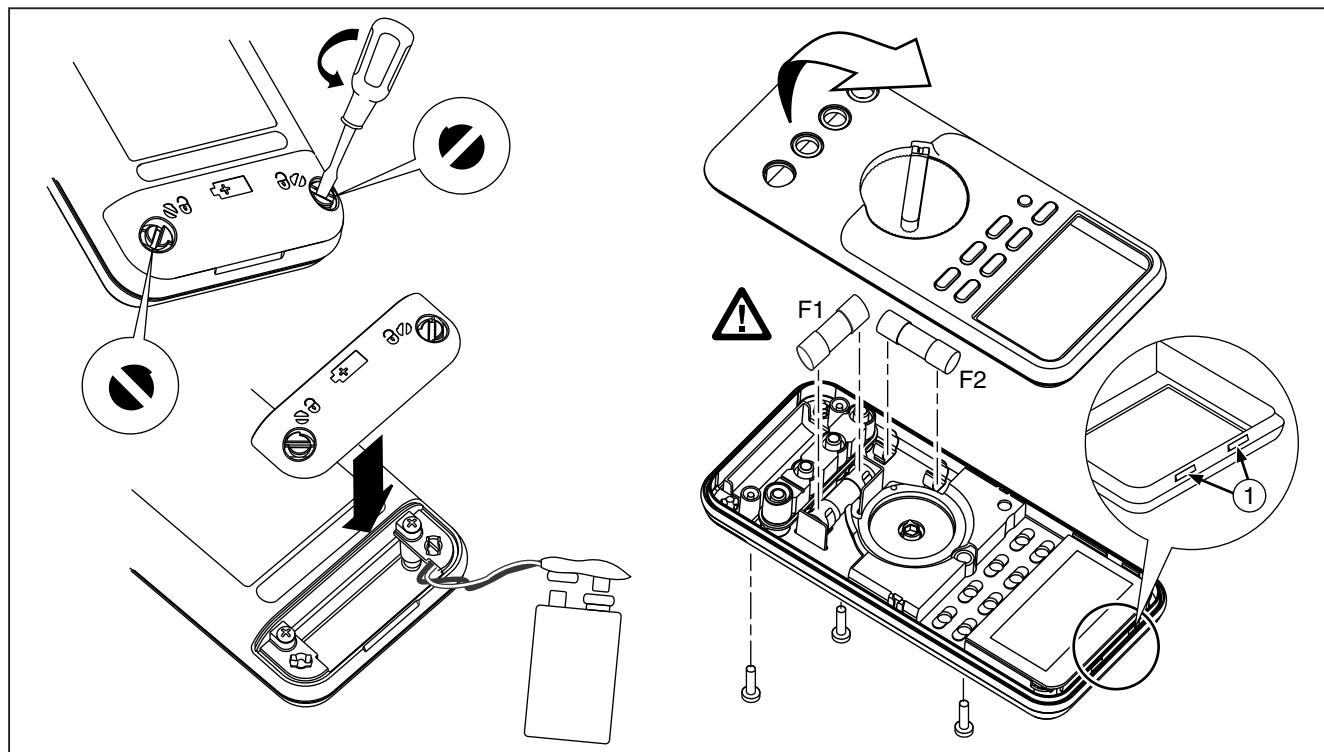
Figura 11. Sostituzione della pila e dei fusibili
