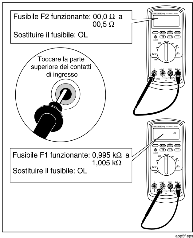
Figura 10. Prova dei fusibili per le misure di corrente
