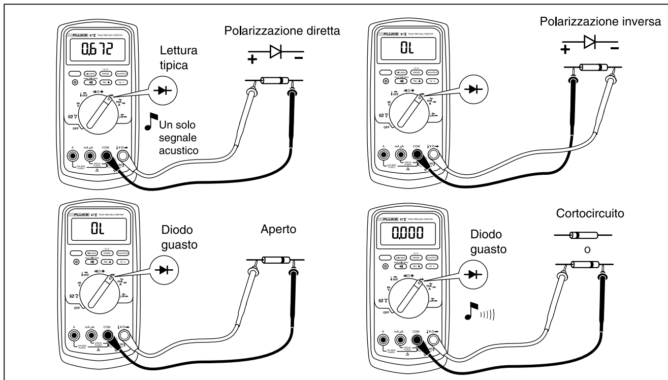
Figura 7. Prova di un diodo
