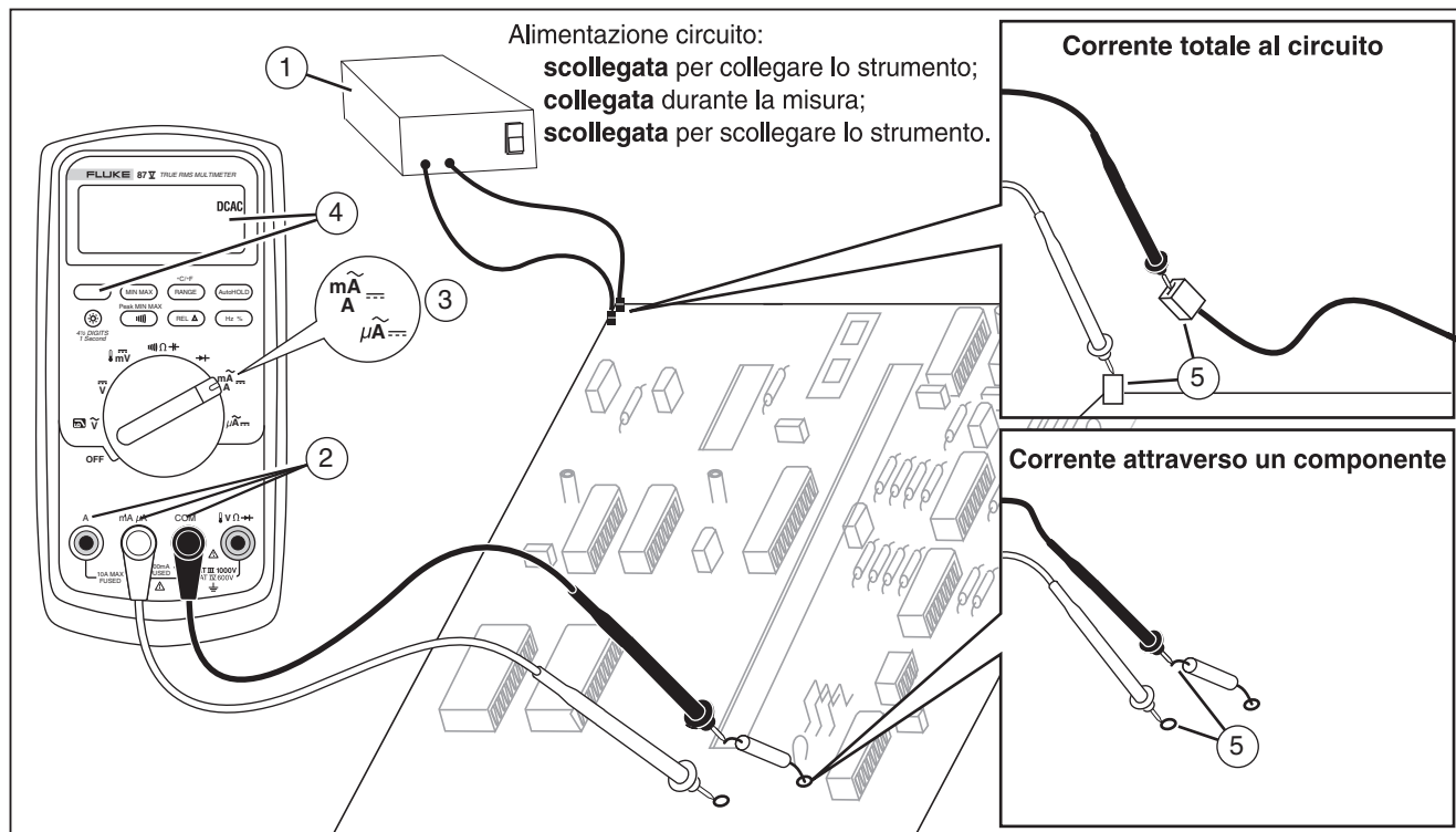
Figura 8. Misura di corrente
