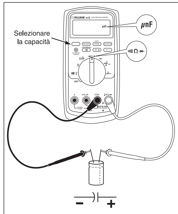
Figura 6. Misura di capacità
