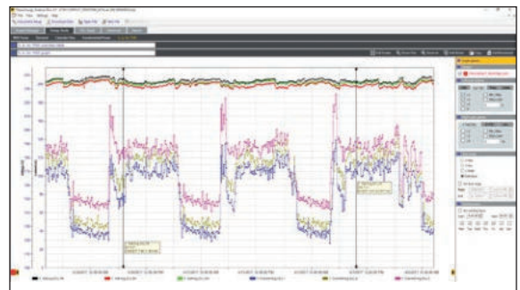
Grafico tendenziale di tensione e corrente.
