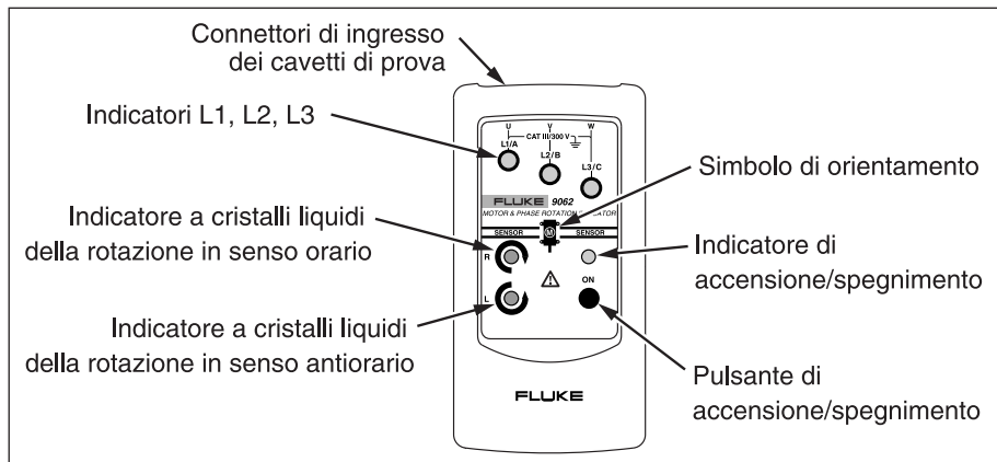
Figura 1. Indicatore di rotazione motore e sequenza fasi 9062
