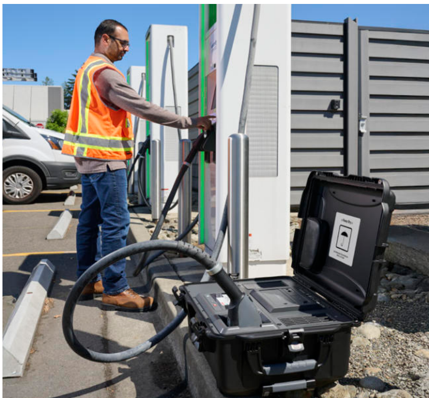
Analizzatore per stazioni di ricarica rapida CC per EV Fluke FEV500
