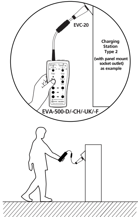
Figure 9: PE pretest
