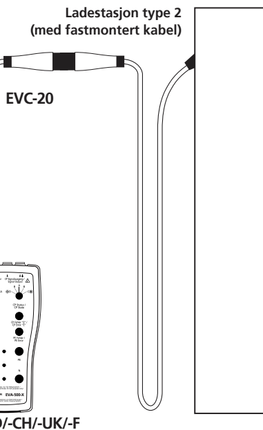
Figur 7: Tilkobling av prøveadapteren til en ladestasjon type 2 med fastmontert kabel og kjøretøykontakt
