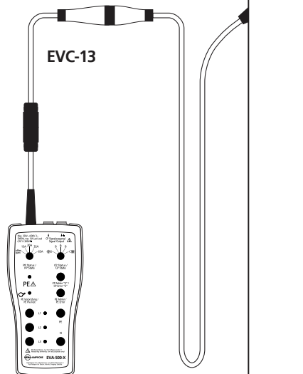
Kuva 8: Testisovittimen liitäntä latausasema tyyppi 1:een, jossa kiinteä kaapeli ja ajoneuvoliitäntä
