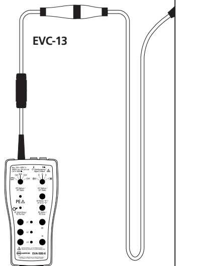
Figura 8: Collegamento dell'adattatore per test a una stazione di ricarica di tipo 1 con cavo fisso e connettore veicolo
