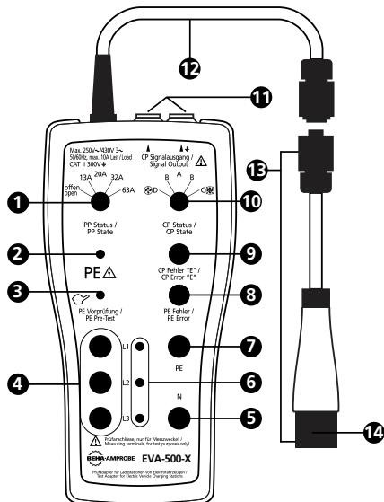
Kuva 2: Testisovittimen käyttöelementit ja liittimet
