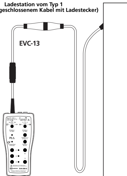
Abbildung 8: Anschluss des Prüfadapters an eine Ladestation Typ 1 mit fest angeschlossenem Kabel mit Ladestecker
