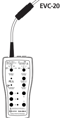
Rysunek 6: Podłączenie adaptera testowego do stacji ładowania typu 2 z gniazdem wyjścia mocowanym na panelu
