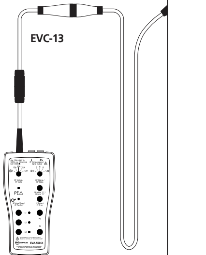
Rysunek 8: Podłączenie adaptera testowego do stacji ładowania typu 1 z kablem podłączonym na stałe i złączem pojazdu
