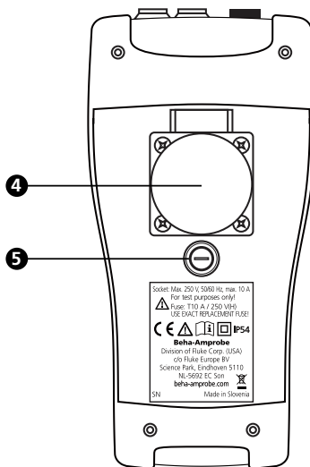
Kuva 4: Testisovittimen taustapuoli
