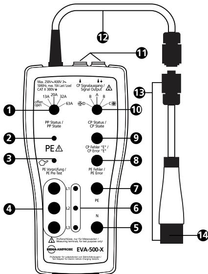
Figura 2: Elementos y conectores de funcionamiento del adaptador de prueba
