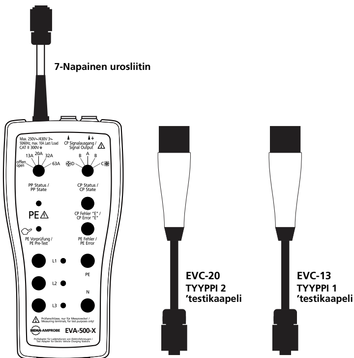
Kuva 5: Käytettävissä olevat testikaapelit testisovitinsarjoille
