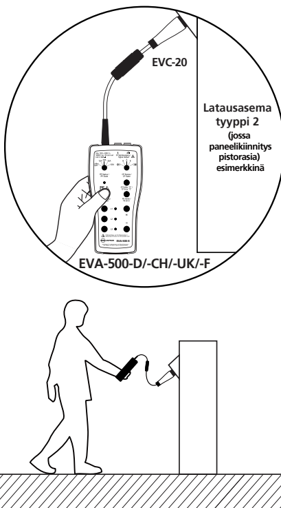
Kuva 9: PE-esitesti
