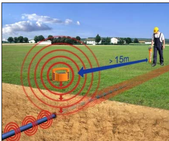
Fig. 7: Uso del trasmettitore in accoppiamento induttivo
