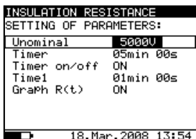
Fig. 18: Setting parameters
