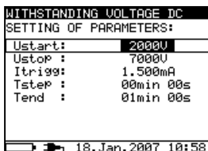
Fig. 45: Setting parameters
