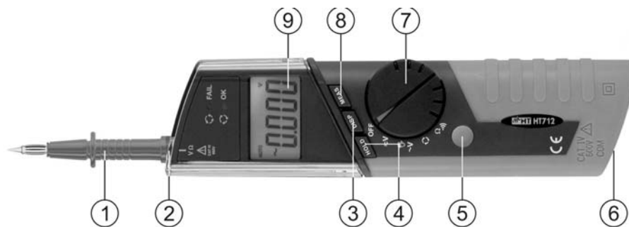
Fig. 1: Descrizione dello strumento
