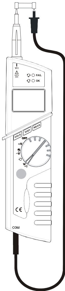
Fig. 7: Misura di resistenza e test continuità
