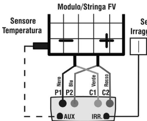
Fig. 7a: Collegamento strumento al modulo/stringa FV
