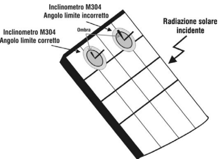
Fig. 7b: Posizionamento inclinometro M304
