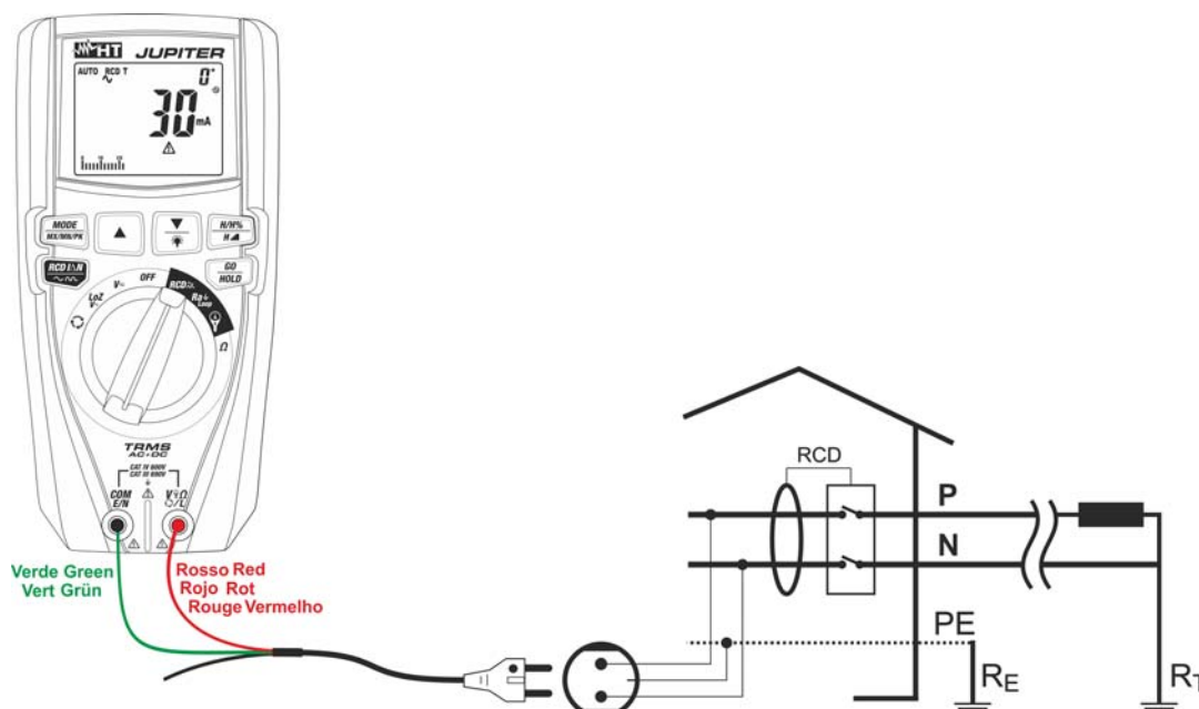
Fig. 29: Uso dello strumento per test RCD su sistema Monofase con cavo a spina Schuko
