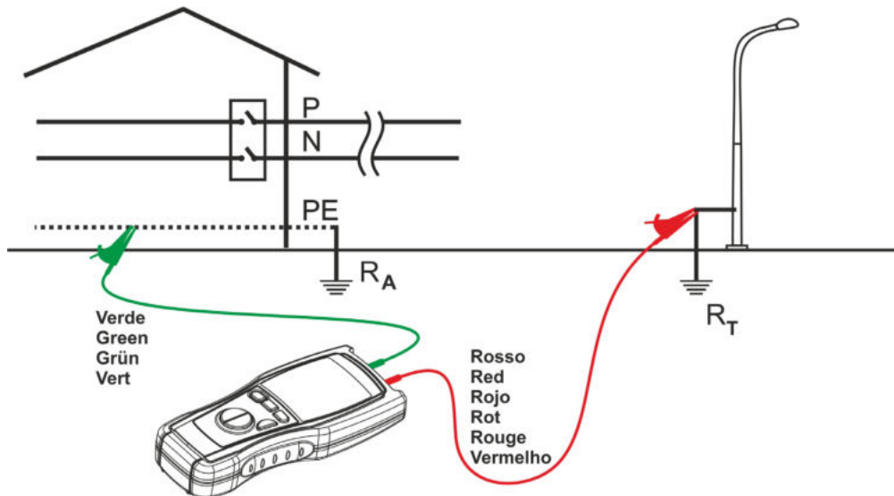
Fig. 3: Esempio di connessione dello strumento per la misura di Terra a 2 Punti
