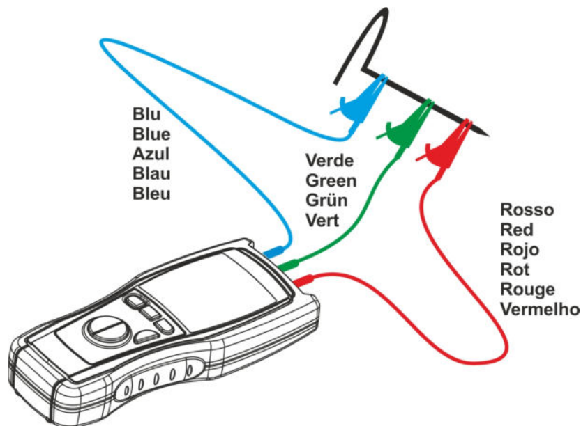
Fig. 5: Connessioni dello strumento per l'azzeramento dei cavi in modalità EARTH-3P
