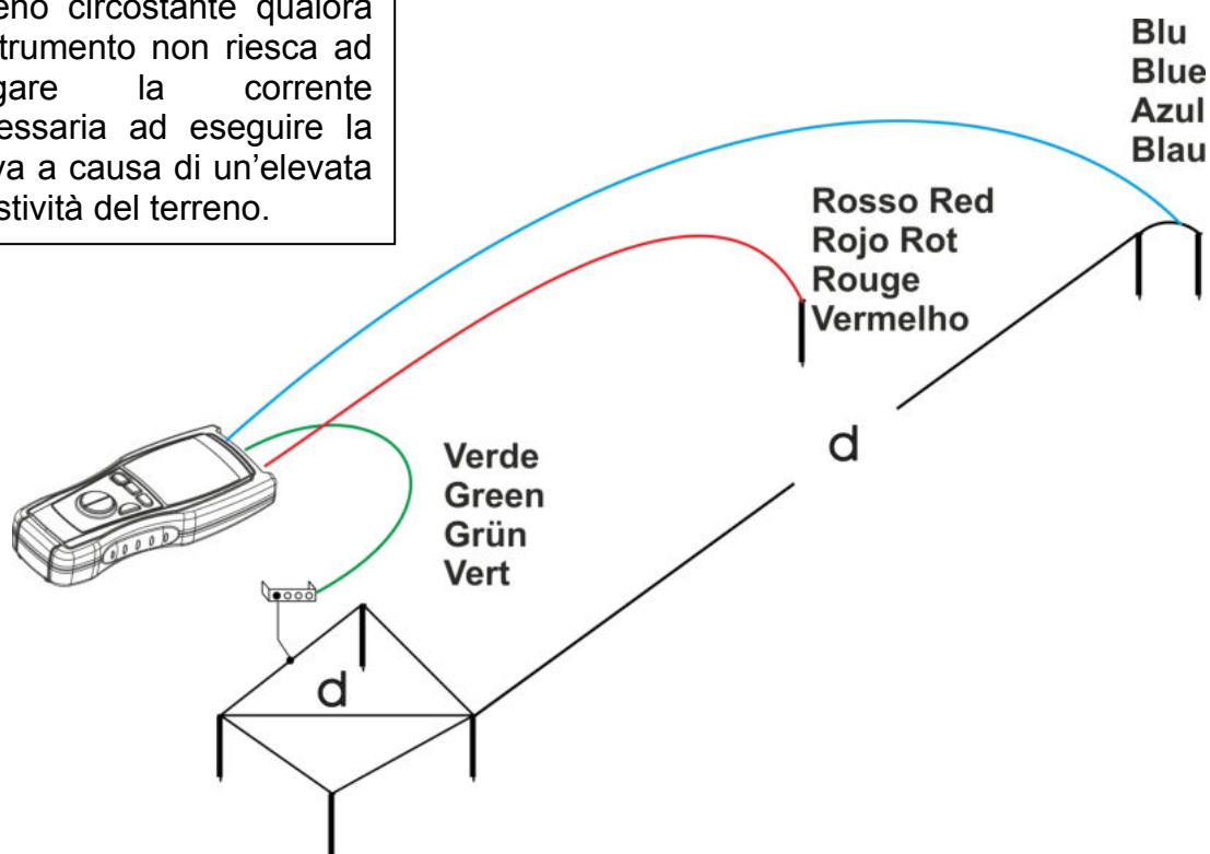
Fig. 8: Misura resistenza di terra per dispersori di medie e grandi dimensioni
