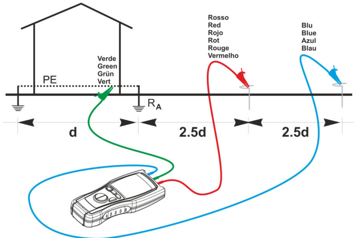
Fig. 6: Connessione dello strumento per la misura di Terra a 3 Punti
