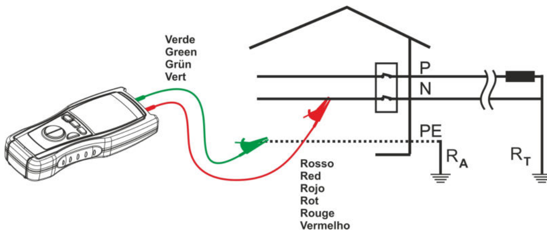
Fig. 4: Esempio di connessione dello strumento per la misura di Terra a 2 Punti (utilizzabile solo per sistemi TT).
