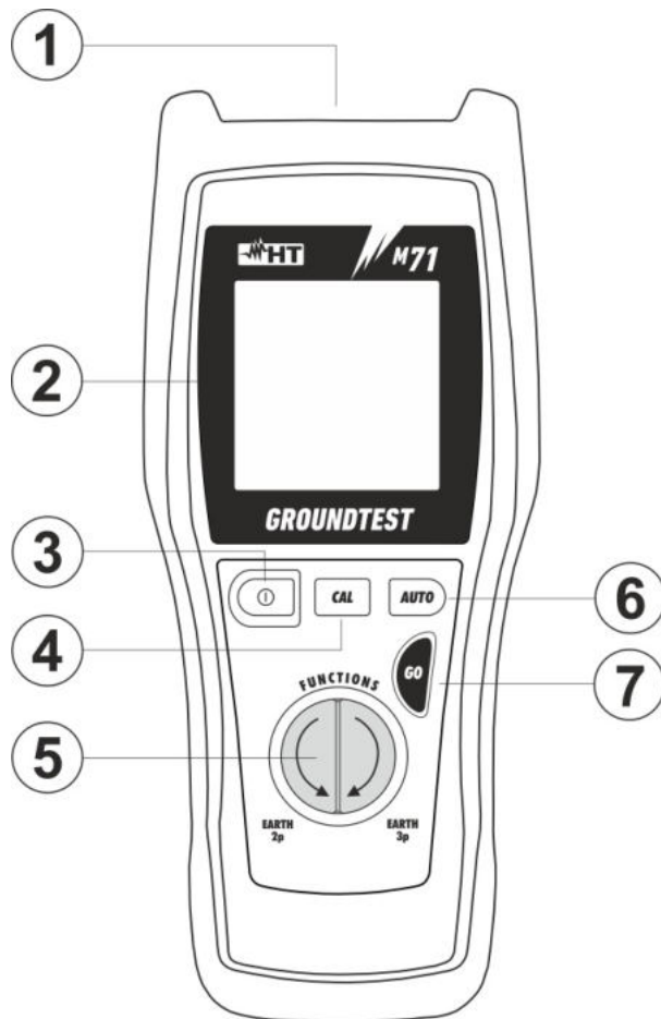
Fig. 1: Descrizione dello strumento
