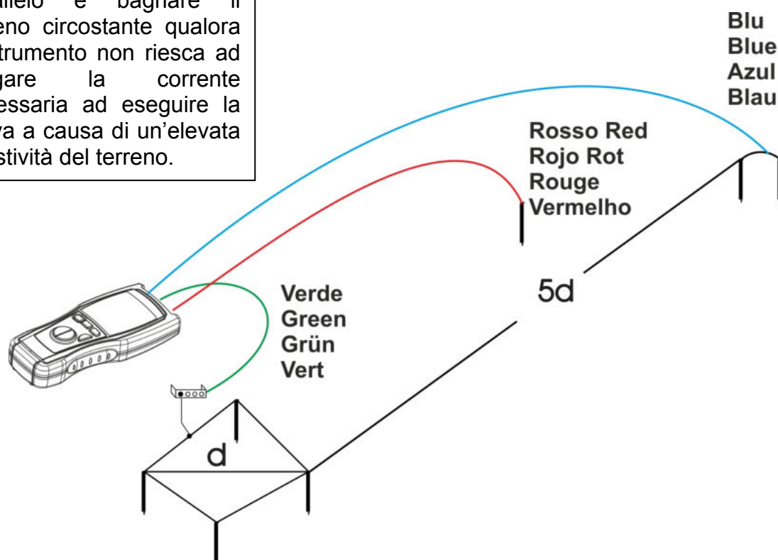
Fig. 7: Misura della resistenza di terra per dispersori con piccole dimensioni
