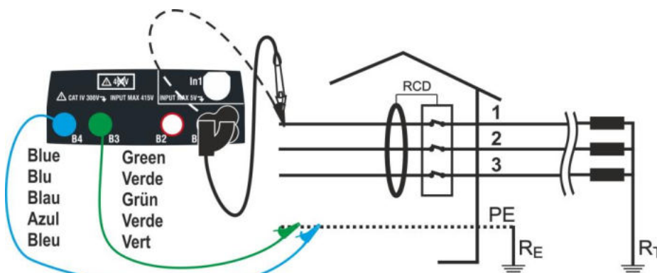
Fig. 16: Collegamento in sistema trifase 400V+ PE (no N) con cavi singoli e puntale remoto (no RCD tipo B)
