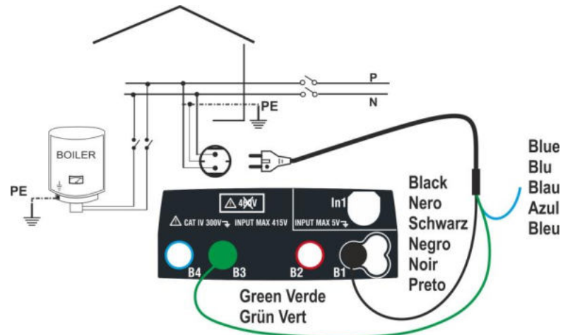
Fig. 9: Verifica dell'isolamento L-PE tramite spina shuko
