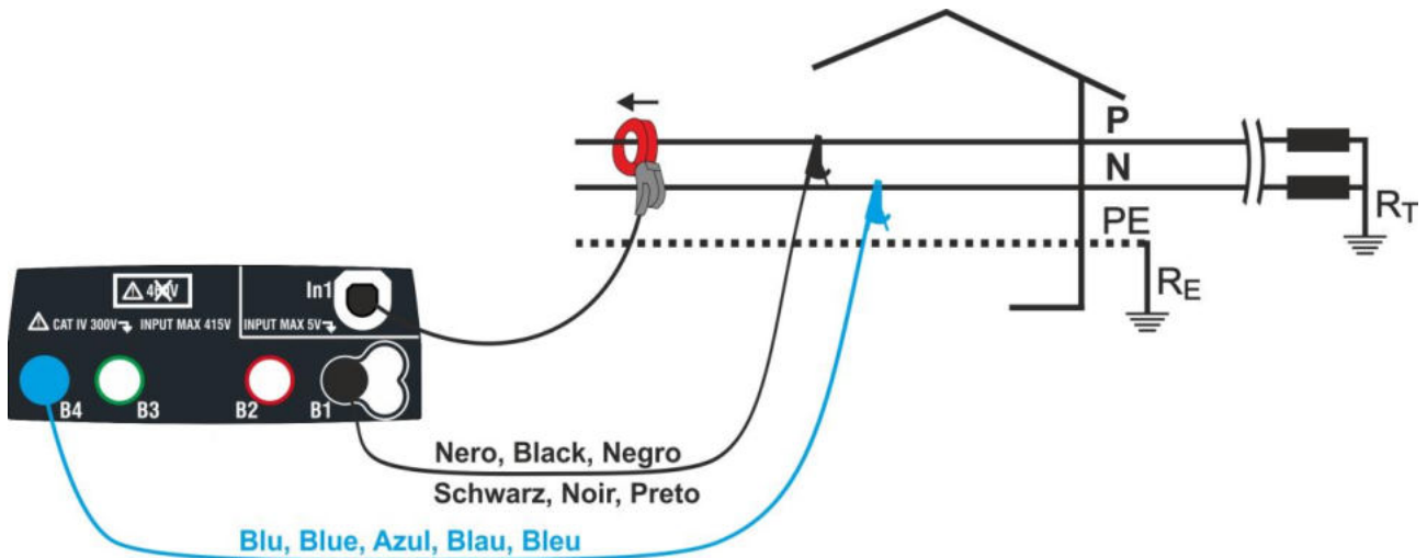
Fig. 36: Collegamento per misura su impianto Monofase
