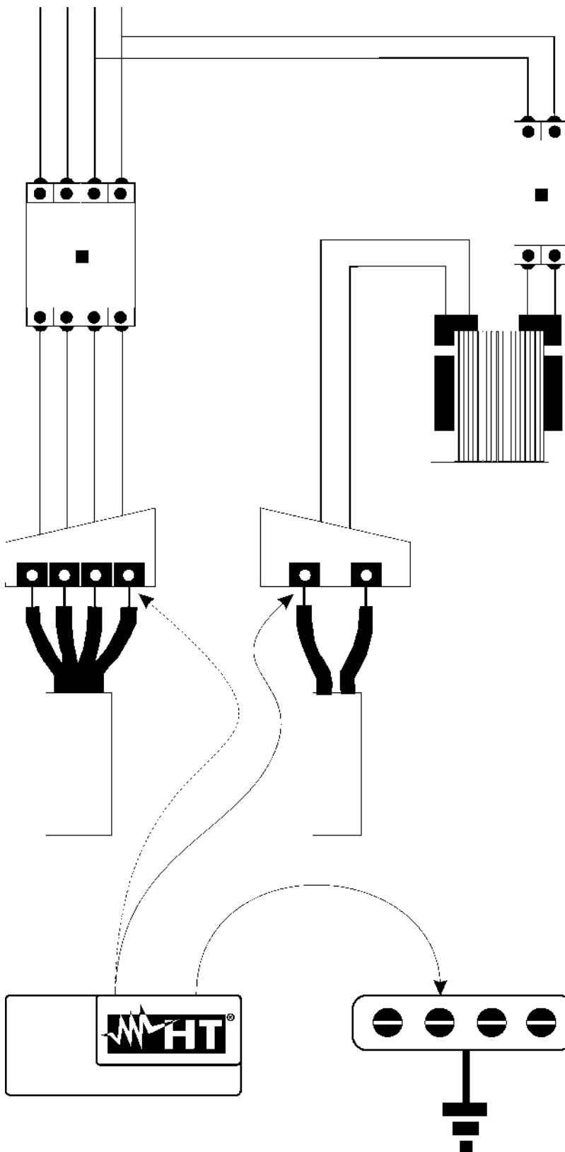
Fig. 45: Misure di separazione tra circuiti in un impianto
