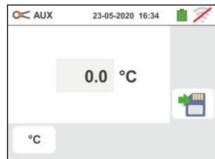
Fig. 33: Misura parametri ambientali con sonde esterne
