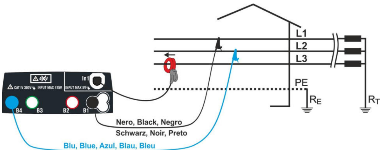
Fig. 37: Collegamento per misura su impianto Trifase equilibrato
