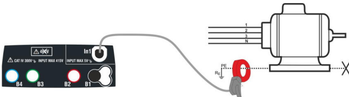
Fig. 27: Misurazione diretta della corrente di dispersione in impianti trifase
