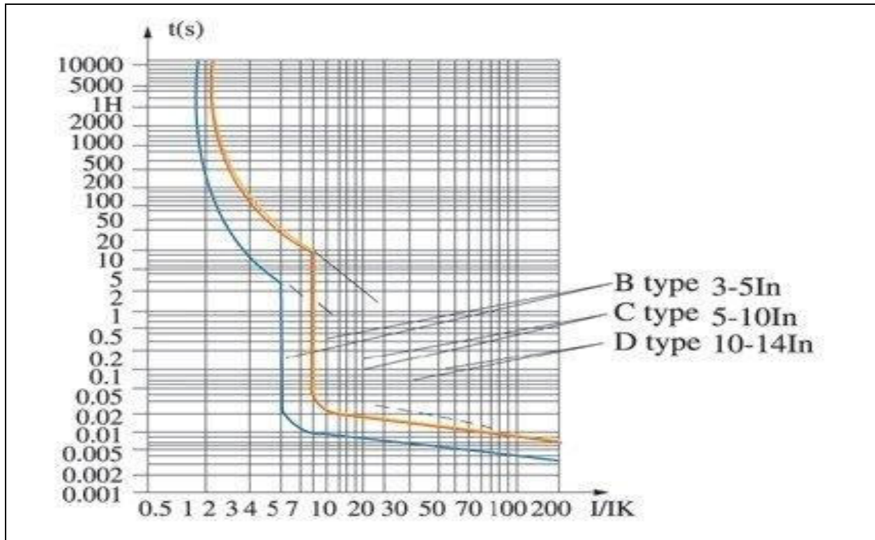
Fig. 46: Esempio di curve di intervento protezioni magnetotermiche (MCB)
