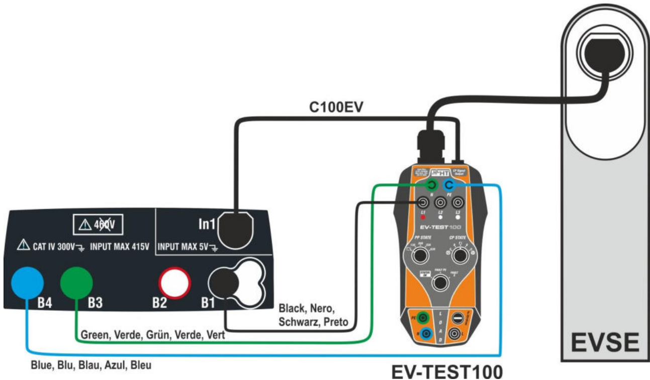
Fig. 38: Collegamento dell'adattatore EV-TEST100 allo strumento e al sistema EVSE
