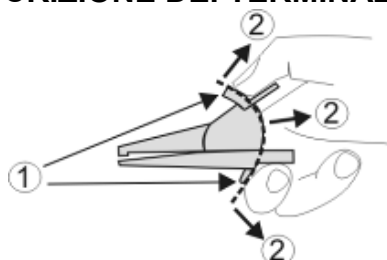
Fig. 4: Descrizione dei terminali di misura
