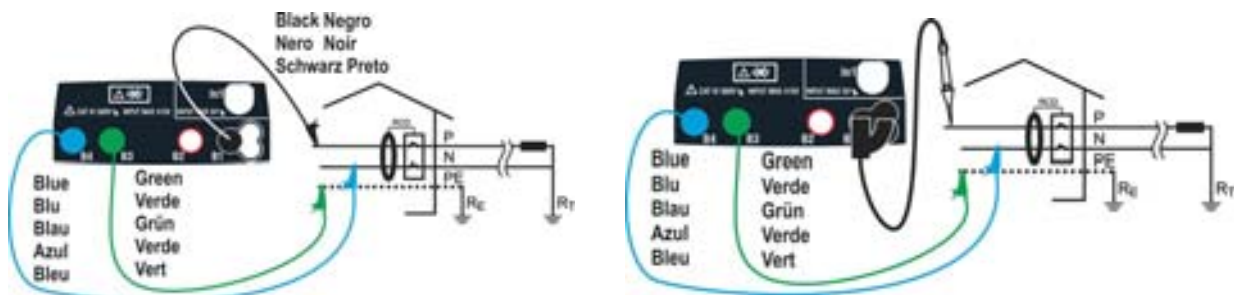
Fig. 13: Collegamento in sistema monofase 230V con cavi singoli e puntale remoto
