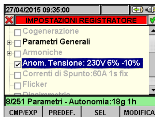
Fig. 65: Videata Anomalie di Tensione
