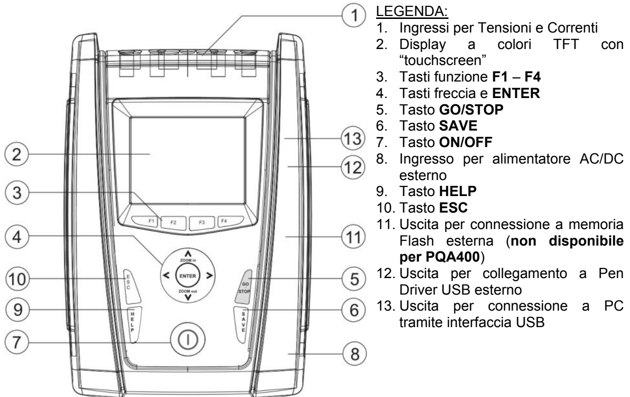
Fig. 1: Descrizione parte frontale dello strumento
