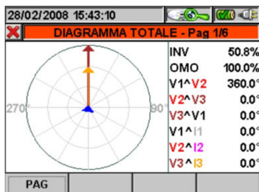
Fig. 109: Diagramma vettoriale totale in sistema Trifase 4-fili
