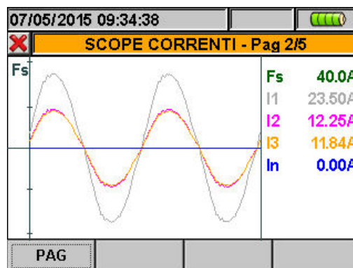
Fig. 29: Videata forme d'onda delle correnti per sistema trifase 4-fili
