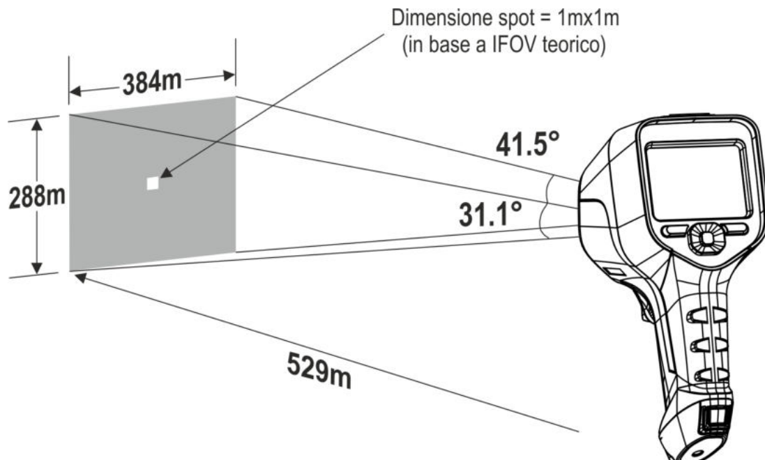
Fig. 48: Rappresentazione del campo visivo FOV dello strumento
