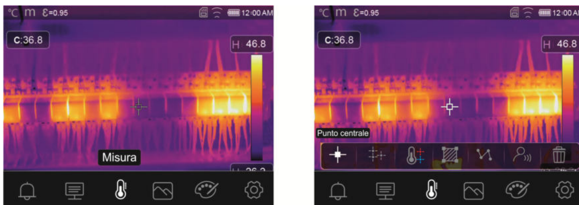
Fig. 33: Menu Misura
