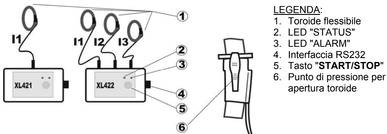
Fig. 1: Descrizione dello strumento
