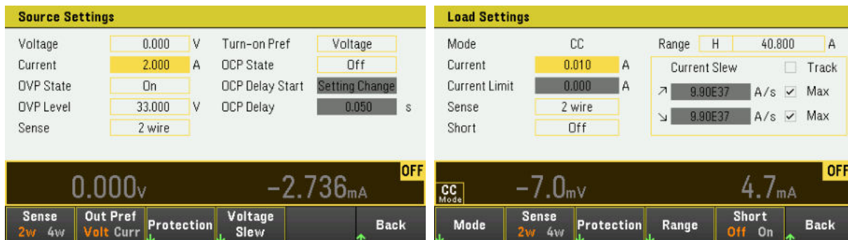
Mode alimentation
