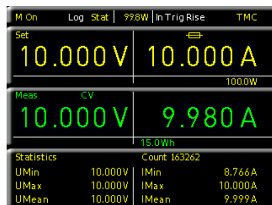
Fig. 4.1 Display values R&S®HMC8041
