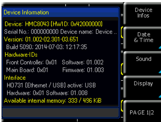
Abb. 9.3: Geräteinformation
