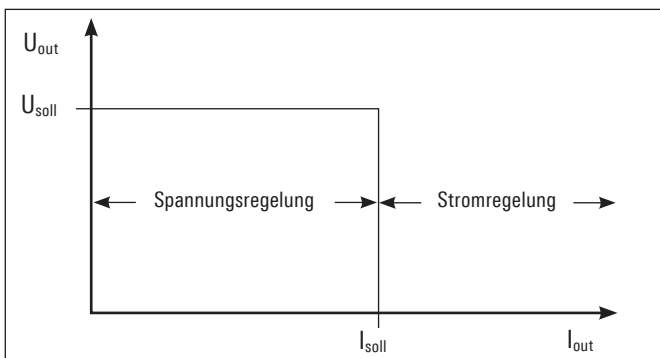
Abb. 5.1: Strombegrenzung
