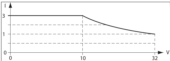
Abb. 4.4: R&S®HMC8043 Leistungshyperbel
