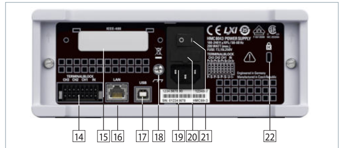
Abb. 2.2: Geräterückseite R&S®HMC8043
